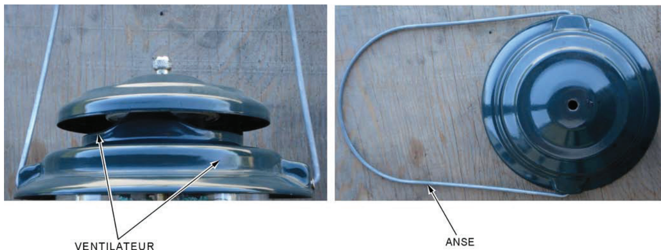
Figure 11-9-5 Ensemble ventilateur et anse
